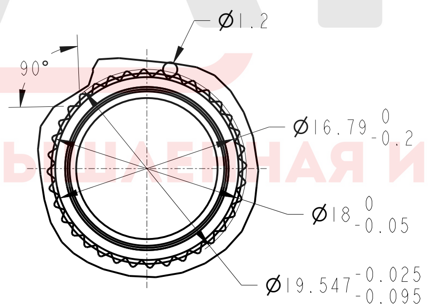
截面 C-C 比例 3.000
